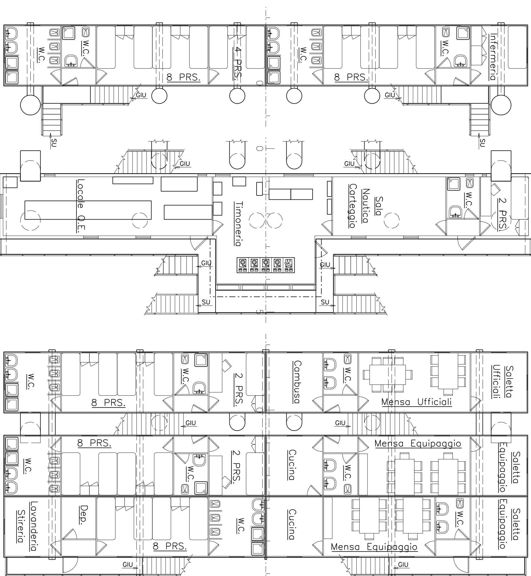
SOVRASTRUTTURA 1° LIVELLO
